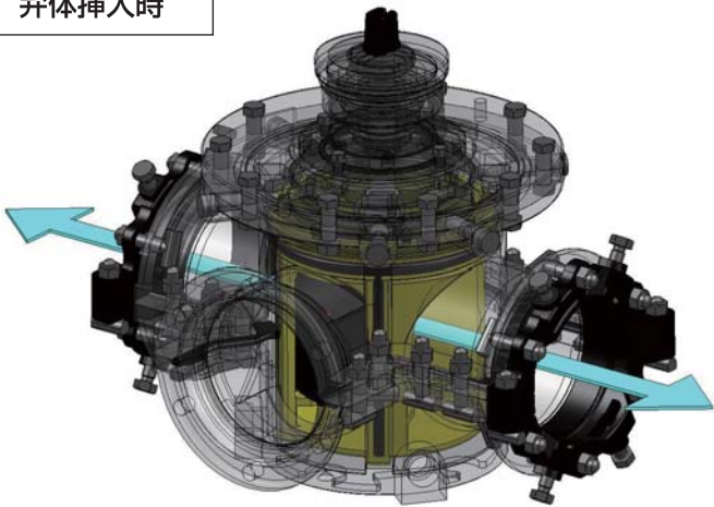
弁体挿入時
